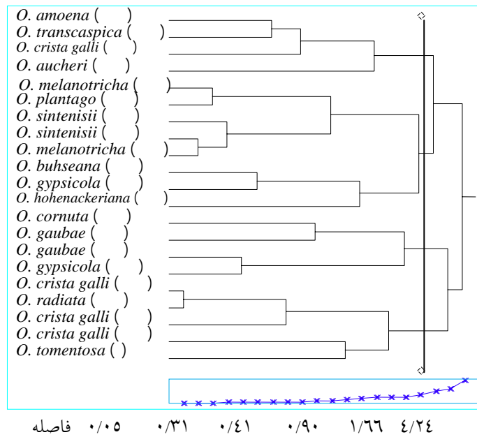
شکل ۵- دندروگرام حاصل از تجزیه کلاستر به روش Ward بر اساس دو پارامتر A_1 و A_2
