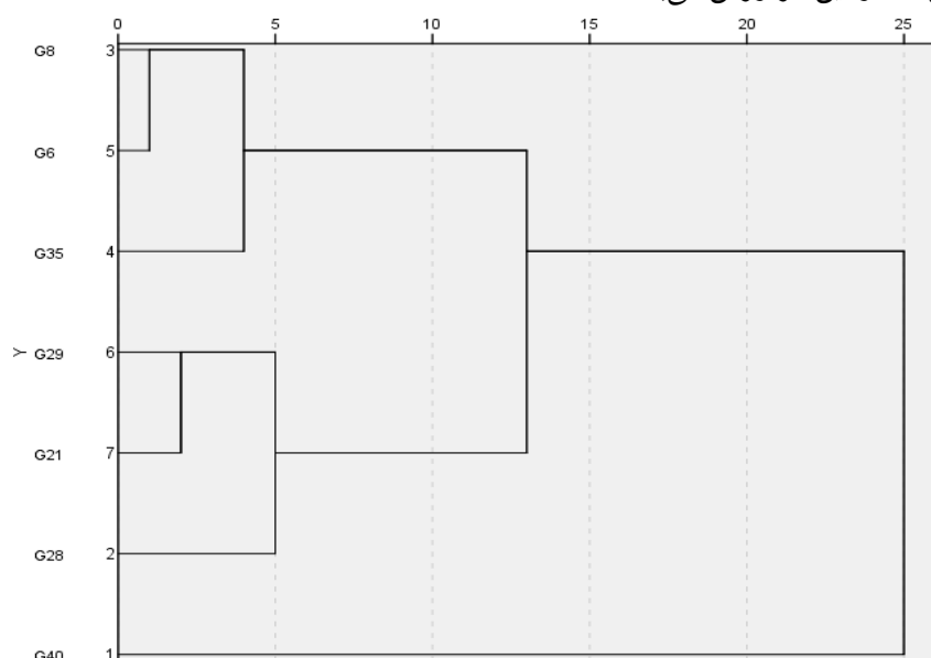
شکل ۴- دندروگرام حاصل از تجزیه خوشه‌ای به روش میانگین فاصله بین جفت نمونه‌ها روی ۷ ژنوتیپ منتخب دیم بر مبنای میانگین
