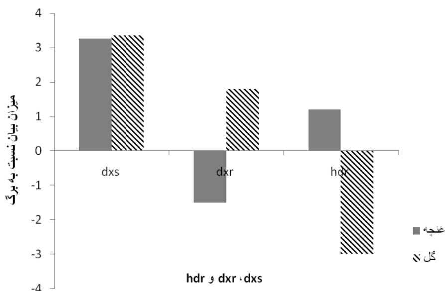
شکل ۳- مقایسه بیان ژن‌های DXS ، DXR و HDR در غنچه و گل نسبت به برگ
