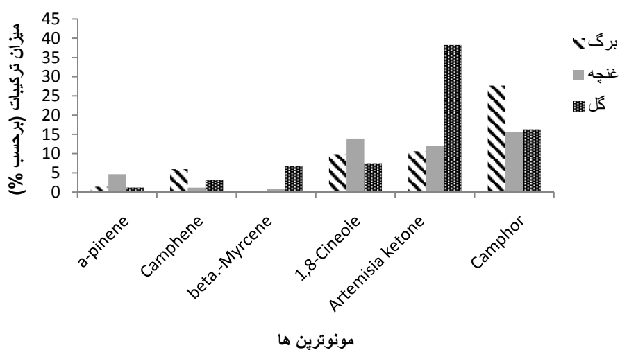
شکل ۲- درصد اصلی‌ترین مونوترپن‌های تشکیل‌دهنده اسانس گیاه Artemisia annua
